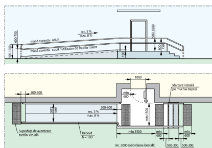
Fig. V.32.2 Rampă de acces paralelă cu intrare în clădire
