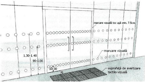
Fig. V.23. – Exemplu de conformare a suprafețelor vitrate în cadrul foi de ușă și realizarea contrastului vizual
