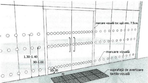
Fig. V.24. – Exemplu de conformare a suprafețelor vitrate în cadrul foii de ușă și realizarea contrastului vizual, atunci când ușa și suprafețele adiacente sunt vitrate
