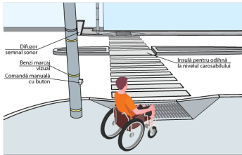
Fig. RE14.a Traversarea străzilor cu lățime mai mare pe 4 benzi de circulație. Perspectivă
