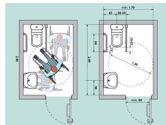
Fig. V42a Amenajarea unei cabine WC adaptate - tip B
