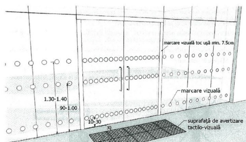
Fig. V.23. – Exemplu de conformare a suprafețelor vitrate în cadrul foii de ușă și realizarea contrastului vizual
